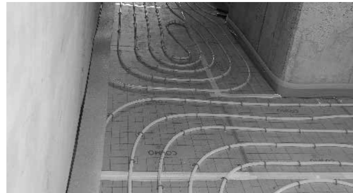
13.04.2023 – Einbau der Leitungen für die Fussbodenheizung in den Umkleide- und Nebenräumen.
